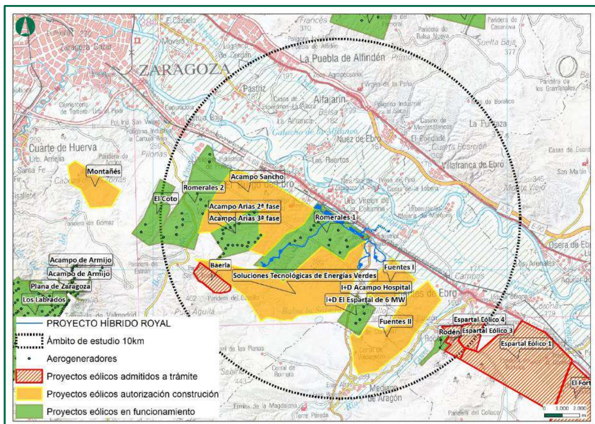
Figura 57. Parques eólicos en el ámbito de estudio (10 km). Fuente: ICEARAGON y elaboración propia.
