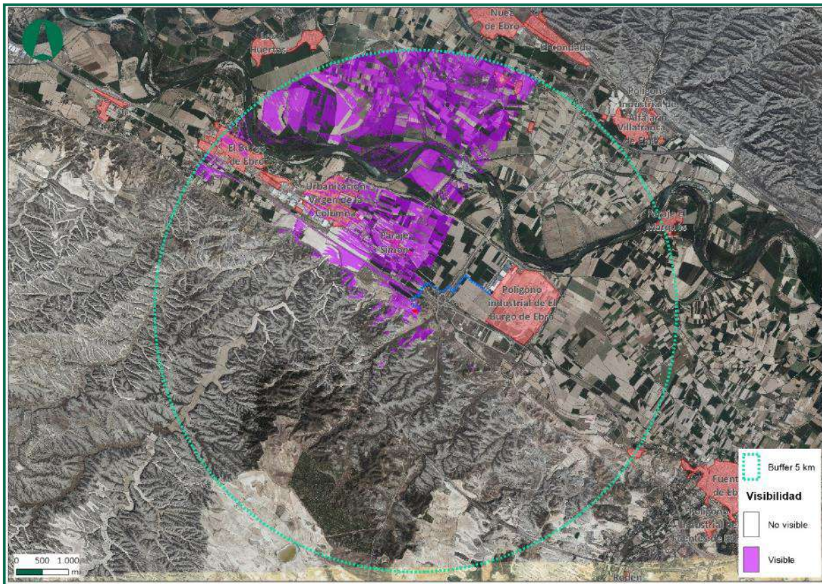
Figura 39. Visibilidad de la SET en una cuenca visual de 5 km. Fuente: Elaboración propia.
